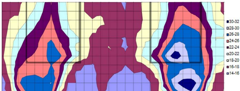
Figura 1. Gráfico de distribución de isotermas en uno de los paramentos del salón de rectores. Nótese que el mayor gradiente térmico se produce en los cuadros (sombra rectangular) ubicados encima de los calefactores.
