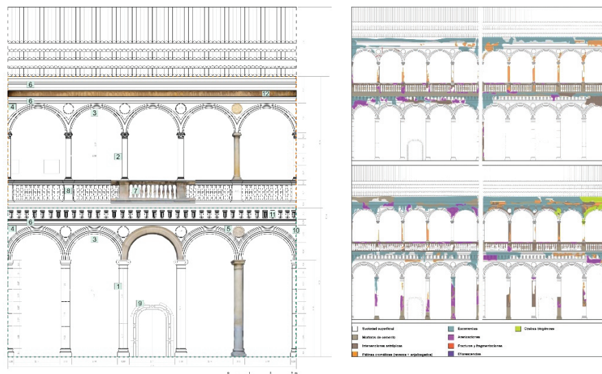
Figura 1. Detalle de alzado Noreste y mapa de alteraciones en los cuatro alzados del Patio de la Capilla-UGR.
